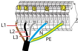
Borne côté Backup Box (triphasé)
