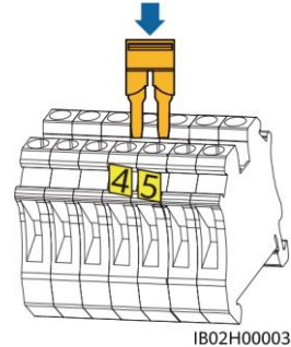
Borne CA du réseau électrique X2(monophasé/triphasé)
