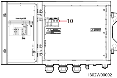
(10) Commutateur de charge hors réseau
