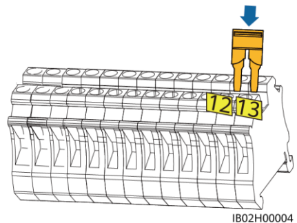
Borne CA de l'onduleur X3 (triphasé)
