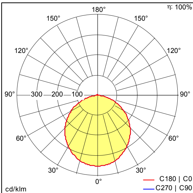
D36865AA_ONDA2_P_D1150_LED22000-840.ltd
