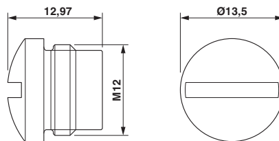
Dessin coté
