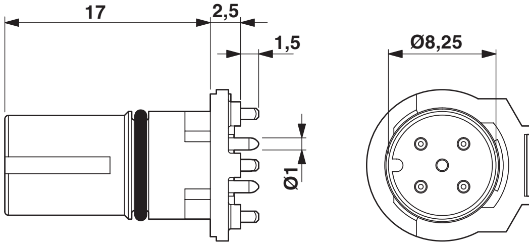
Dessin coté
