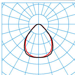
ArimoFit M73 PW19 30-840 ET TX370098 ■ C0 - C180 ■ C90 - C270 UGR I = 16,7 UGR q = 16,7 DIN 5040: A50 UTE: 1,00 C CEN Flux Code: 64 89 97 100 100 0 0 0 0
