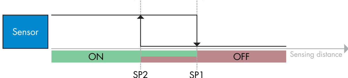
Esempio di rilevamento di presenza – con logica non invertita
