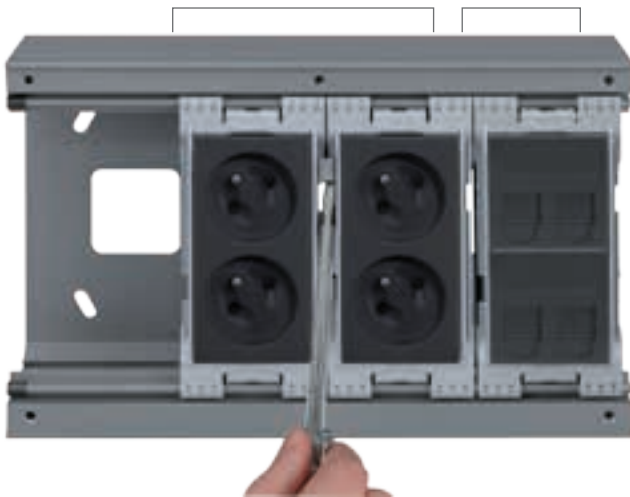
Bloc électrique Bloc V&D
