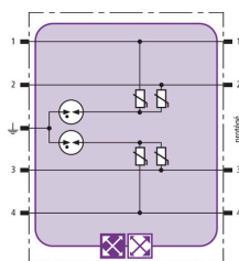
Schéma de principe du circuit BXT ML4 MY 110
