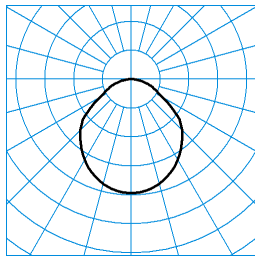
OnplanaAct D11 OTA25 4000 ETDD8 01 (ActDSU) TX299841 ■ C0 - C180 ■ C90 - C270 UGR I = 22,4 UGR q = 22,4 DIN 5040: A40 UTE: 1,00 D CEN Flux Code: 52 83 96 100 100 0 0 0 0
