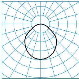
OnplanaAct D11 OTA25 4000 ETDD8 01 (ActDCW) TX299817 ■ C0 - C180 ■ C90 - C270 UGR I = 22,4 UGR q = 22,4 DIN 5040: A40 UTE: 1,00 D CEN Flux Code: 52 83 96 100 100 0 0 0 0
