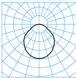
OnplanaAct D11 OTA25 4000 ETDD8 01 (ActDWW) TX299866 ■ C0 - C180 ■ C90 - C270 UGR I = 22,4 UGR q = 22,4 DIN 5040: A40 UTE: 1,00 D CEN Flux Code: 52 83 96 100 100 0 0 0 0
