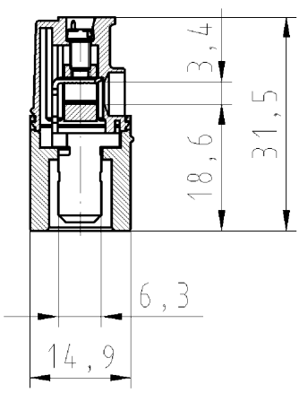
Schnitt A-A section A-A
