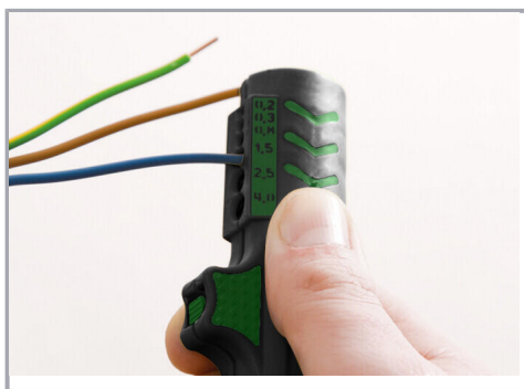
Dénudage du conducteur
