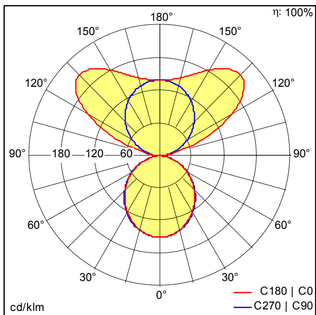
D42843AA+D44967AA_SLOIN_SLIM_ID_840_L2500_PC_WH.Idt
