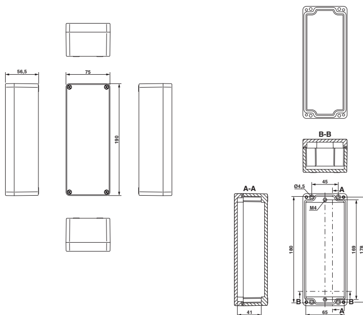
Dessin coté
