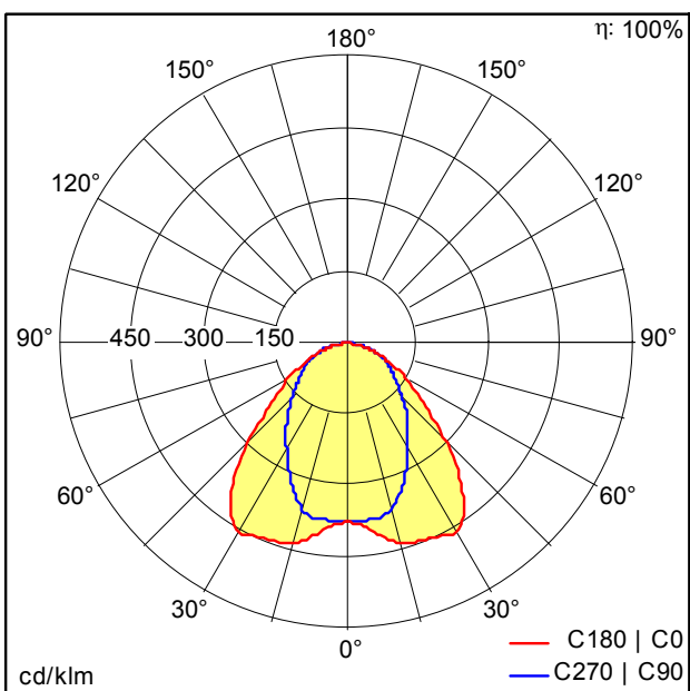
D41246AA_TECTON_C_LED5200-840_L1000_VWB_LDE_WH.Idt
