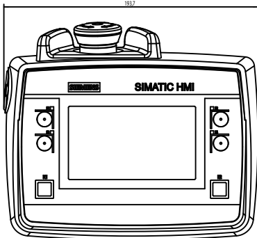
Vorne / Front
