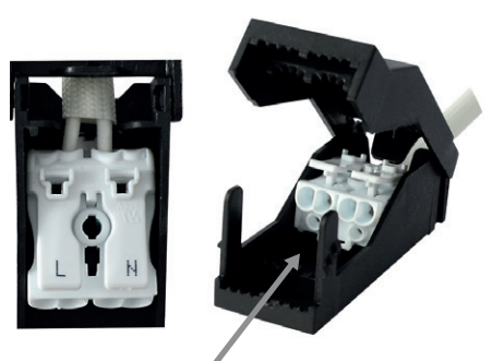
DOUBLE CONNECTION CLIPSABLE POUR MONTAGE EN SÉRIE ( sans outils)
