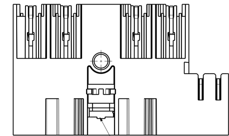
VKMU nur für MSF-Varianten / square nut only for MSF-variants
