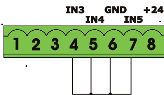
Connexion d'aucun dispositif de sécurité et stop
