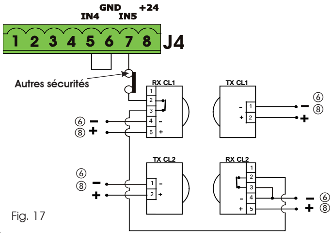
Connexion d'une paire de photocellules en ouverture
