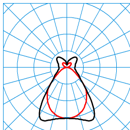
E-Line 7751 HE PMW19 40-840ETDD L150 01 TX375097 ■ C0 - C180 ■ C90 - C270 DIN 5040: B42 UTE: 0,72 D + 0,28 T CEN Flux Code: 60 83 93 72 100 26 59 82 28
