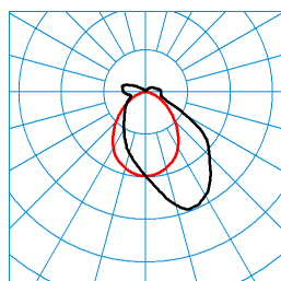
TugraHE Act 12 PAW 50-840 ETDD8 01 (ACTDSU) TX302752 ■ C0 - C180 ■ C90 - C270 DIN 5040: B40 UTE: 0,87 E + 0,13 T CEN Flux Code: 48 79 93 87 100 7 25 60 13
