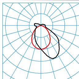
TugraHE Act 12 PAW 50-840 ETDD8 01 (ACTDWW) TX303560 ■ C0 - C180 ■ C90 - C270 DIN 5040: B40 UTE: 0,87 E + 0,13 T CEN Flux Code: 48 79 93 87 100 7 25 60 13
