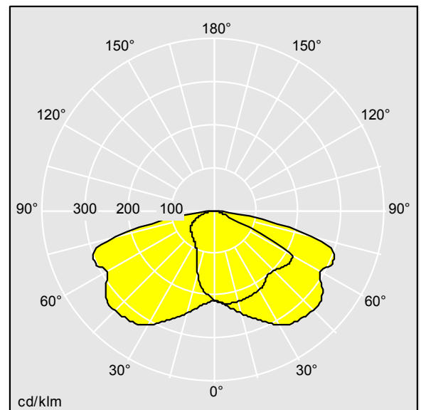
TL_CQL48L50EWC740.lid
