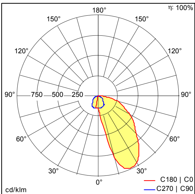
D34983AA_TECTON_C_LED3700-830_L1000_WW_EVG_WH.Idt
