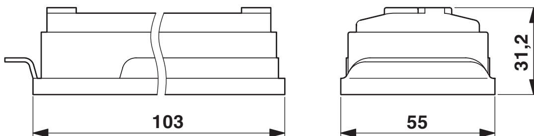
Dessin coté
