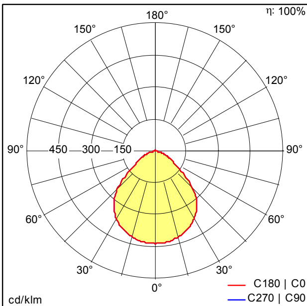
D37457AA_ONDA2_A_LRO_D1150_LED16000-830.ltd
