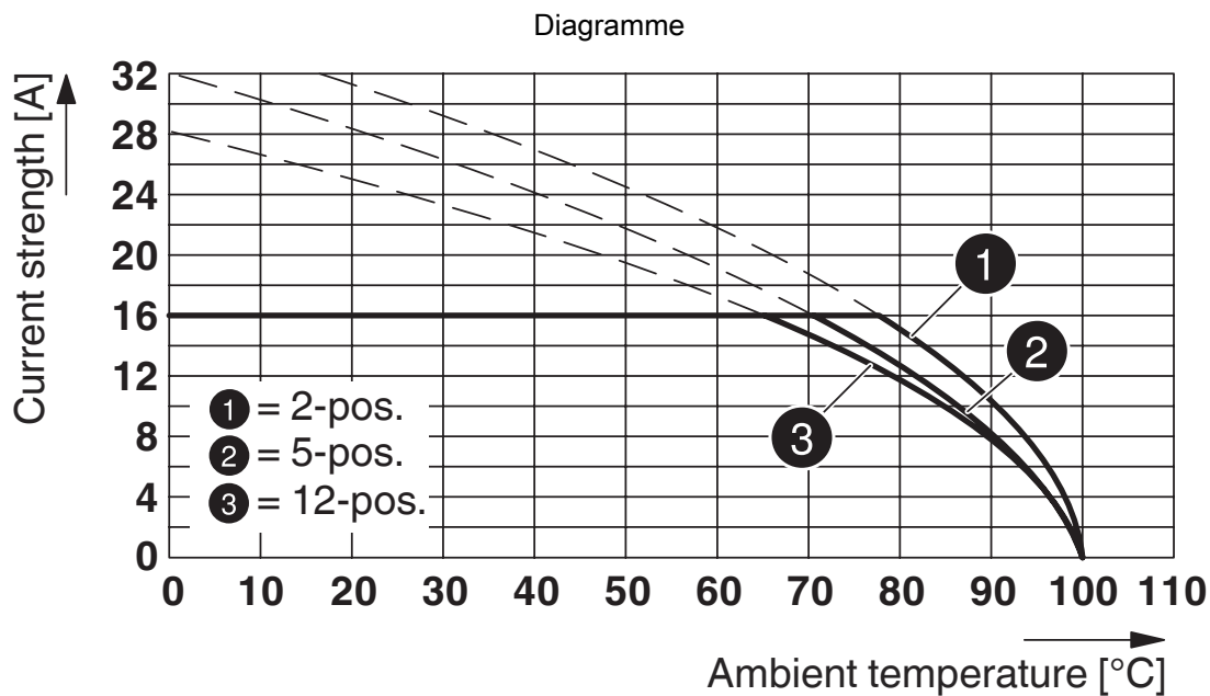
Type : FKIC 2,5 HC/...-ST- 5,08 avec MSTB 2,5 HC/...-ST-5,08
