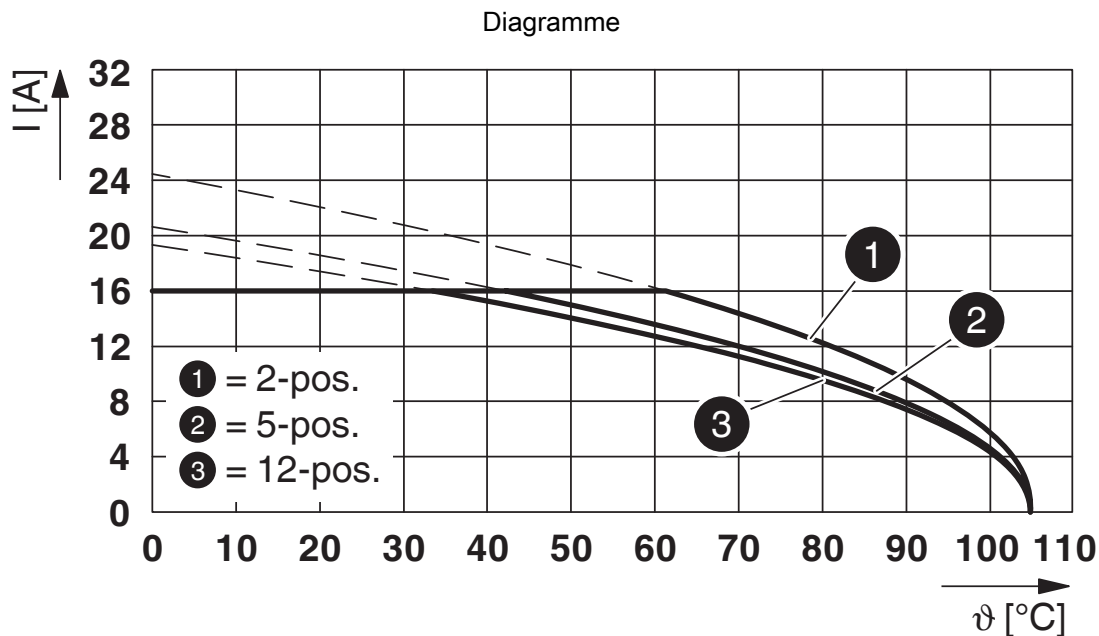
Type : FKIC 2,5 HC/...-ST-5,08 avec IC 2,5 HC/...-G-5,08
