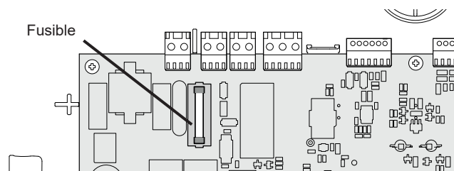
fig. 39 - Remplacement du fusible
