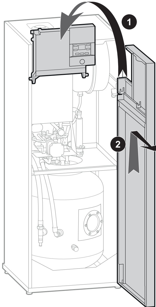
fig. 35 - Dépose de la façade (Perfinox 2 Duo)
