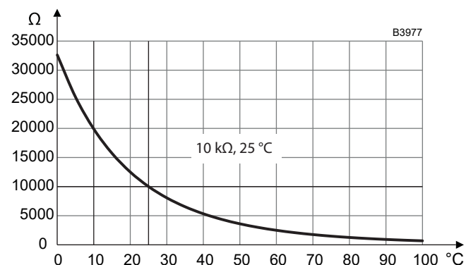
fig. 40 - Valeur ohmique des sondes
