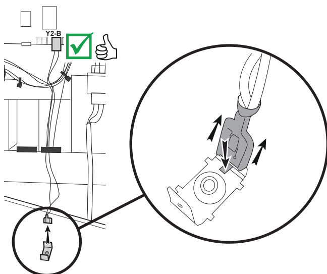
fig. 41 - Perfinox 2 Duo - Débrancher le câble de terre
