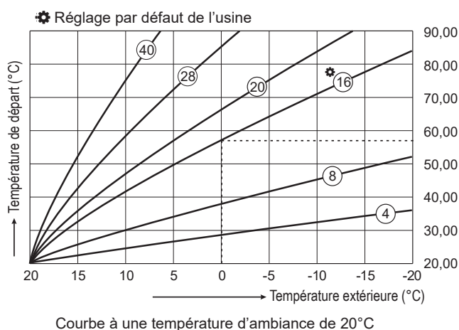
fig. 32 - Courbe de chauffe (Navilink H55)
