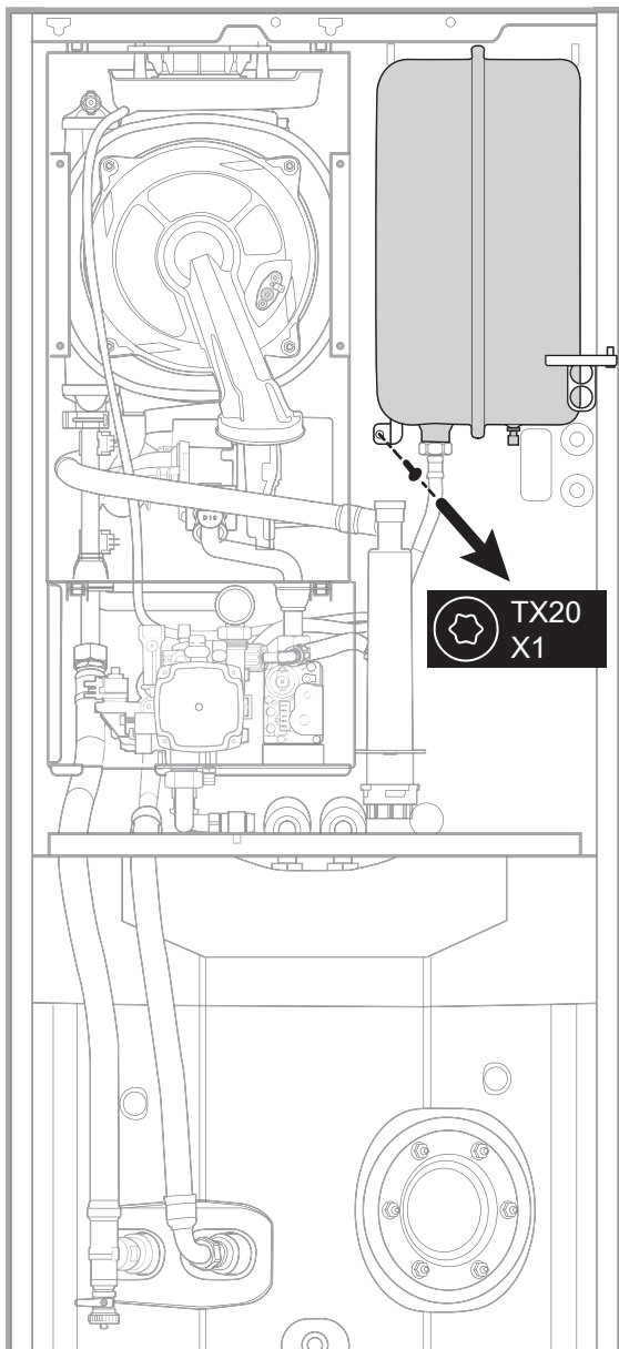
fig. 34 - Dépose du vase d'expansion (Perfinox 2 Duo)
