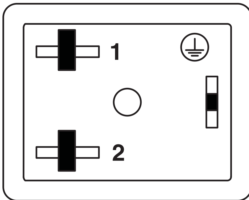
Nombre de pôles connecteur électrovanne, design BI
