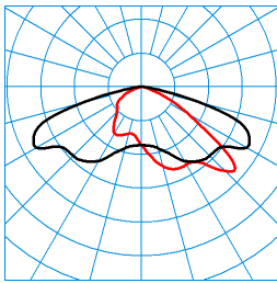
Jovie 70-AB7L-LR/6800-730 8G1 ET TX068616 C0 - C180 C90 - C270 DIN 5040: A30 UTE: 1,00 G CEN Flux Code: 34 71 96 100 100
