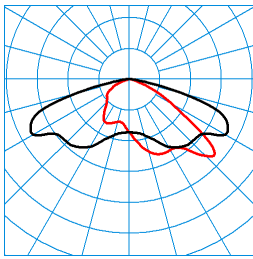
Jovie 70-AB7L-LR/6800-730 8G1 ET (CLO initial value) TX300571 C0 - C180 C90 - C270 DIN 5040: A30 UTE: 1,00 G CEN Flux Code: 34 71 96 100 100
