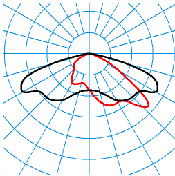
Jovie 70-AB7L-LR/6800-730 8G1 ET (CLO end value) TX301468 C0 - C180 C90 - C270 DIN 5040: A30 UTE: 1,00 G CEN Flux Code: 34 71 96 100 100
