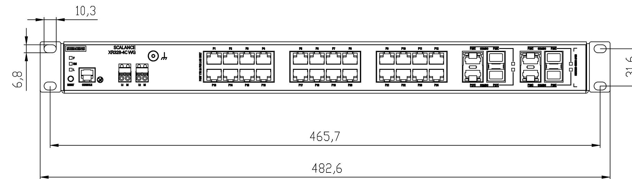
Vorne / Front
