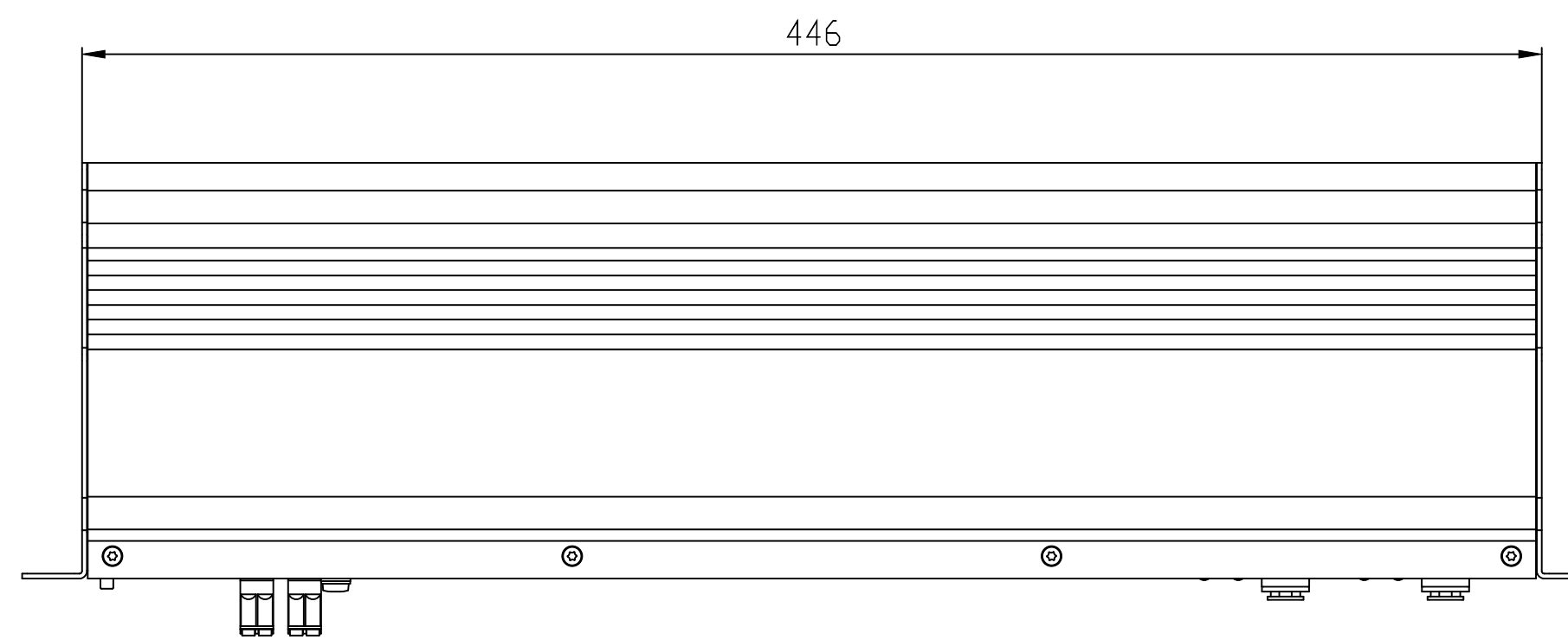
Oben / Top
