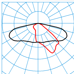
LIQ 50-AB2L-LR/5100-740 6G1S TX054102 DIN 5040: A30 UTE: 1,00 G CEN Flux Code: 36 71 96 100 100
