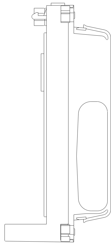
Rechts / Right
