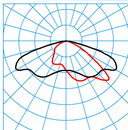
Jovie 70-AB7L-LRA/13500-740 16G1 ET TX076477 ■ C0 - C180 ■ C90 - C270 DIN 5040: A30 UTE: 1,00 G CEN Flux Code: 35 72 97 100 100
