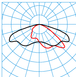
Jovie 70-AB7L-LRA/13500-740 16G1 ET (CLO initial value) TX300641 ■ C0 - C180 ■ C90 - C270 DIN 5040: A30 UTE: 1,00 G CEN Flux Code: 35 72 97 100 100
