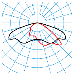
Jovie 70-AB7L-LRA/13500-740 16G1 ET (CLO end value) TX300582 ■ C0 - C180 ■ C90 - C270 DIN 5040: A30 UTE: 1,00 G CEN Flux Code: 35 72 97 100 100
