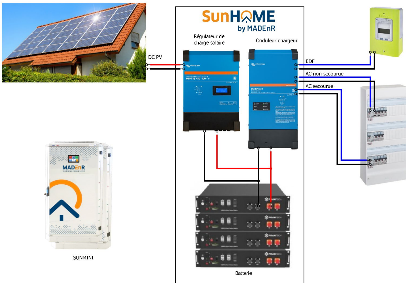
Figure 50 : Schéma de principe de la SunMini
