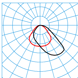
Cultega Act T SMC PAW 600 ETDI KL 05 (ACTDCW) TX280859 ■ C0 - C180 ■ C90 - C270 DIN 5040: A40 UTE: 1,00 D CEN Flux Code: 54 85 97 100 100
