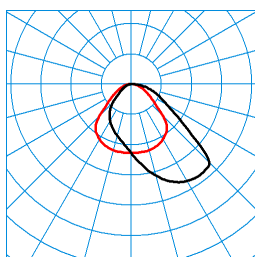
Cultega Act T SMC PAW 600 ETDI KL 05 (ACTDSU) TX280860 ■ C0 - C180 ■ C90 - C270 DIN 5040: A40 UTE: 1,00 D CEN Flux Code: 54 85 97 100 100
