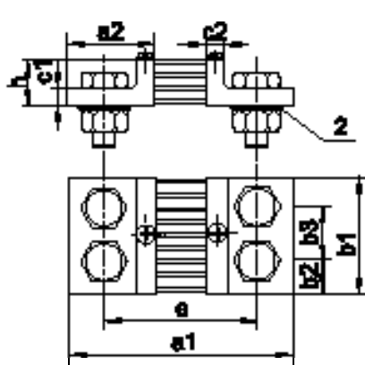
Fig.1. Dimensions de fixation des shunts 1 - base isolante, 2 - rondelle élastique.
