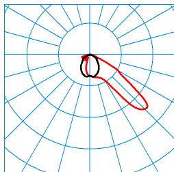
Jovie 50I-AM2L-SLR3/6800-740 6G1 ET (CLO end value) TX300384 ■ C0 - C180 ■ C90 - C270 DIN 5040: A40 UTE: 1,00 F CEN Flux Code: 47 91 100 100 100
