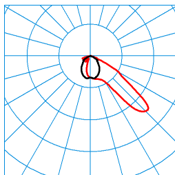
Jovie 50I-AM2L-SLR3/6800-740 6G1 ET (CLO initial value) TX301194 ■ C0 - C180 ■ C90 - C270 DIN 5040: A40 UTE: 1,00 F CEN Flux Code: 47 91 100 100 100
