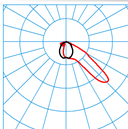
Jovie 50I-AM2L-SLR3/6800-740 6G1 ET TX19524 ■ C0 - C180 ■ C90 - C270 DIN 5040: A40 UTE: 1,00 F CEN Flux Code: 47 91 100 100 100
