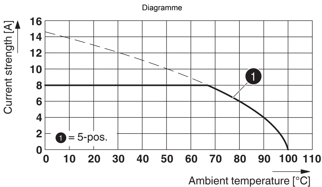
Type : FMC 1,5/... -ST-3,5 avec MCD 1,5/...-G3-3,5 P26 THR MAG
