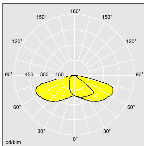
TL_CQL48L50NR740.idt
