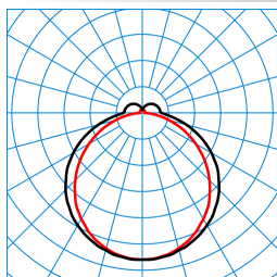
Olisq LWD3 DW 30-840 ETBLE +DMR IP54 IK TX430114
