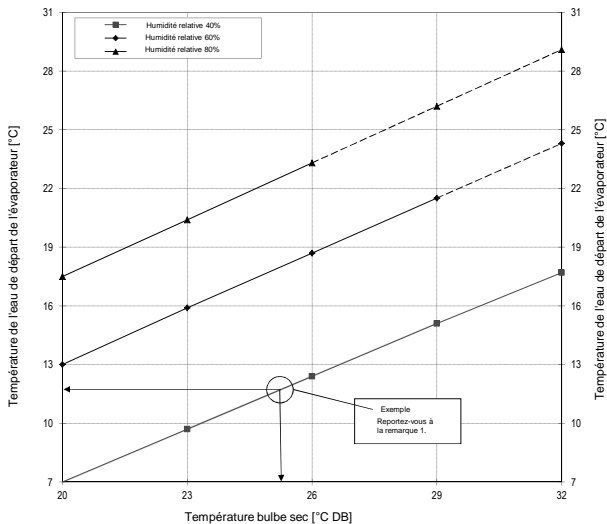
Limite de température de l'eau de départ de l'évaporateur pour éviter la condensation
