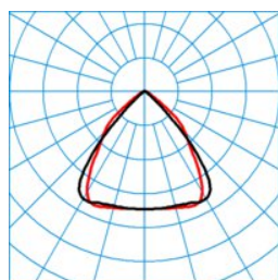
ELINE LW2240-110 ML 830 L150 2 50 ■ C0 - C180
