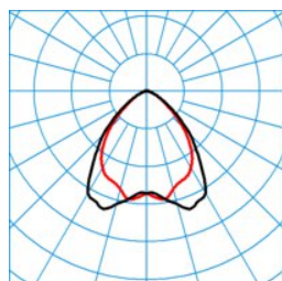
ELINE LW2240-110 ML 830 L150 4 50 ■ C0 - C180
