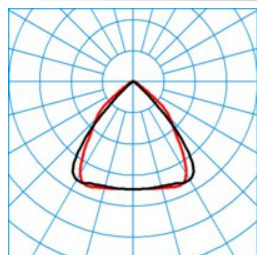
ELINE LW2240-110 ML 830 L150 0 50 ■ C0 - C180
