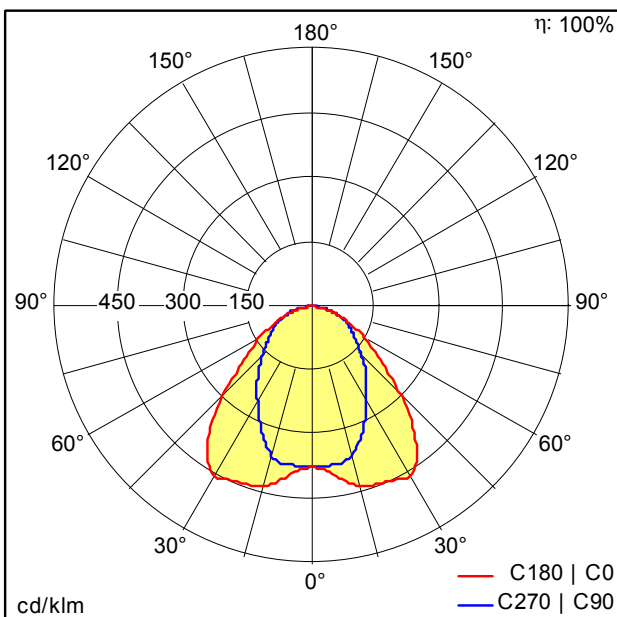
D41246AA_TECTON_C_LED5500-840_L1500_VWB_LDE_BK.ltd
