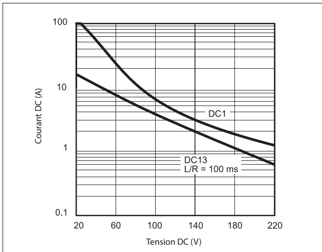
H 68-1 - Pouvoir de coupure maxi pour une charge en DC (68.22/23)
