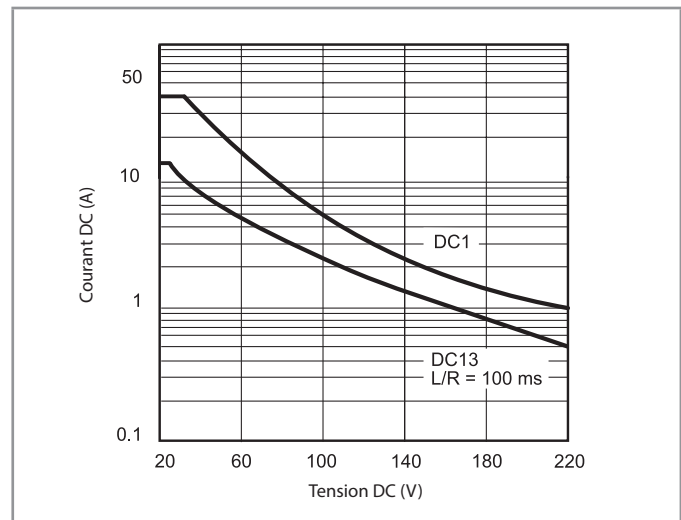
H 68-2 - Pouvoir de coupure maxi pour une charge en DC (68.24/25/54/55)
