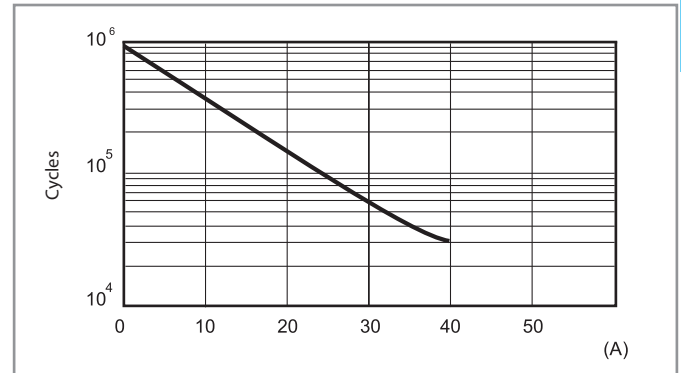
F 68-1 - Durée de vie électrique en fonction de la charge (AC1/AC7a) (68.24/25/54/55)
