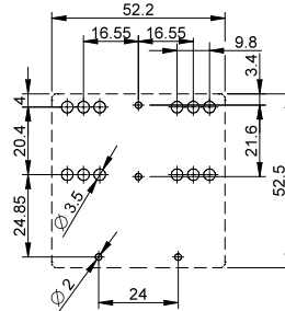
Vue coté cuivre
