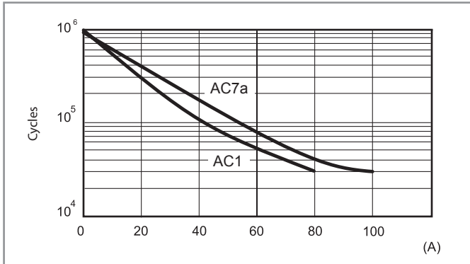
F 68 - Durée de vie électrique en fonction de la charge (68.22/23)
