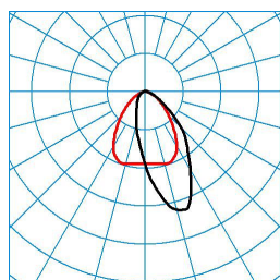
ELINE HE LAN80 840 L225 4 20 DIN 5040 3 = A50 UTE 3 = 0,98 C + 0,02 T CEN flux code = 63 89 98 98 100 0 6 44 2
