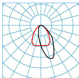
ELINE HE LAN80 865 L225 3 20 DIN 5040 2 = A50 UTE 2 = 0,98 C + 0,02 T CEN flux code = 63 89 98 98 100 0 6 44 2
