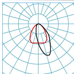
ELINE HE LAN80 827 L225 2 20 DIN 5040 = A50 UTE = 0,98 C + 0,02 T CEN flux code = 63 89 98 98 100 0 6 44 2
