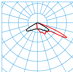
LnPlus 40-AM19L-LR/3200-722 4G1 ET (CLO initial value) TX377678 ■ C0 - C180 ■ C90 - C270 DIN 5040: A30 UTE: 1,00 J CEN Flux Code: 28 76 99 100 100
