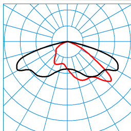
Jovie 70-AB7L-LRA/10000-740 8G1 ET TX068623 ■ C0 - C180 ■ C90 - C270 DIN 5040: A30 UTE: 1,00 G CEN Flux Code: 34 71 96 100 100
