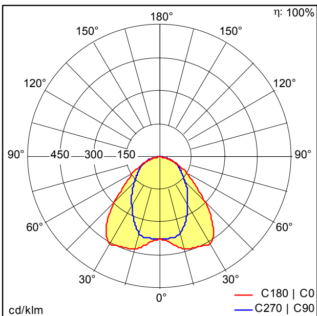
D41246AA_TECTON_C_LED3700-865_L1000_VWB_LDE_SR.Idt
