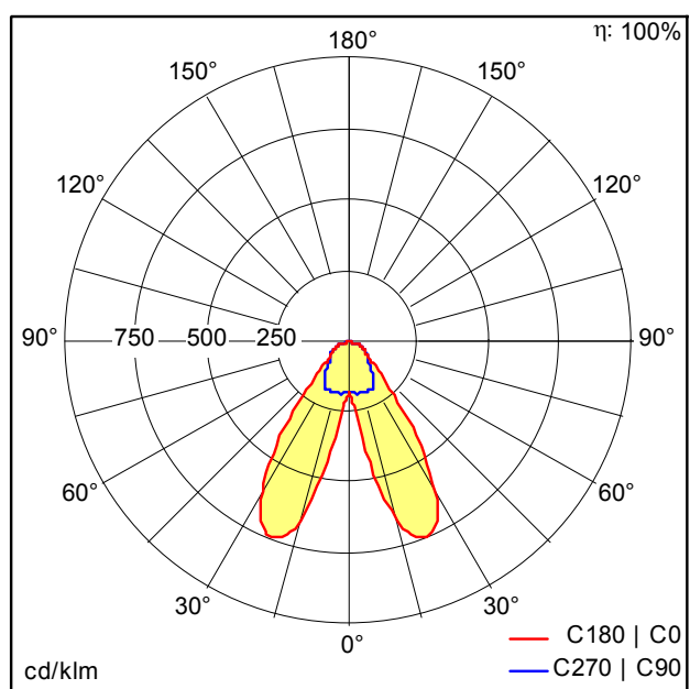
D43655AA_TECTON_C_LED8000-830_L1500_SB_LDE_WH.Idt
