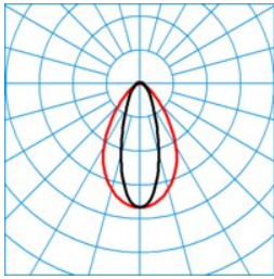
7850 PN35-110 ML 840 L150 12 50
