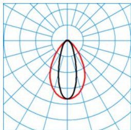
7850 PN35-110 ML 840 L150 14 50
