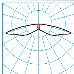
Jovie 50-SB3L-LRA/1350-730 2G1 ET TX068588 ■ C0 - C180 ■ C90 - C270 DIN 5040: A20 UTE: 1,00 l CEN Flux Code: 29 61 91 100 100
